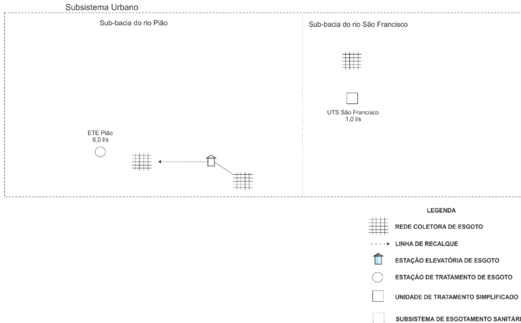
Figura 14 – Esquema com a concepção do Sistema de Esgotamento Sanitário Urbano da unidade de planejamento Pião.
