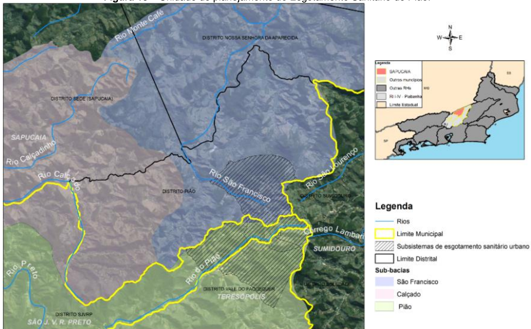
Figura 13 – Unidade de planejamento do Esgotamento Sanitário de Pião.
