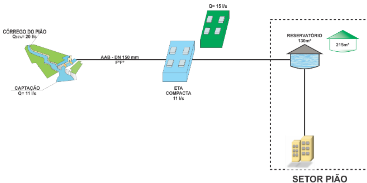
Figura 6 – Esquema do Sistema de Abastecimento de Água proposto para a unidade de planejamento de Pião – metas de curto prazo a serem implementadas até 2019.
