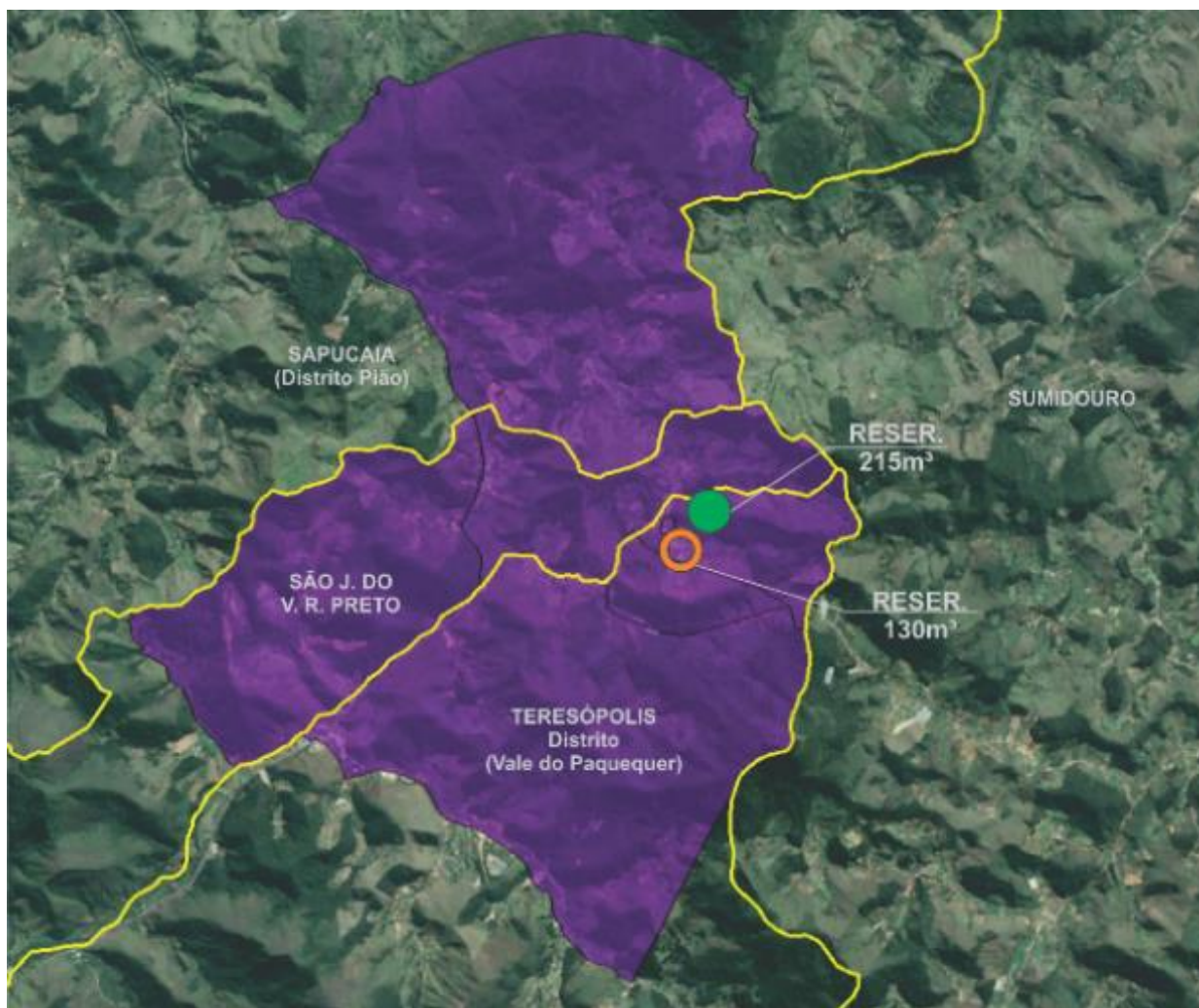
Figura 5 – Localização dos reservatórios existente e a construir ao longo do período do Plano e área de abrangência estimada.
